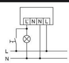
Standarddrift med ekstra konstantlysfunktion med ekstern afbryder.
