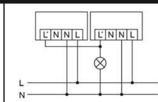
Parallelkobling med maks. 8 sensorer
