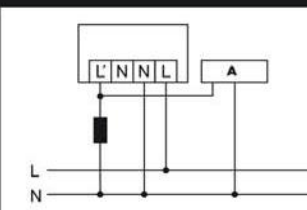
Ved kobling med induktive enheder (f.eks. relæer, kontaktorer, forkoblingsenheder) kan det være hensigtsmæssigt at anvende et RC-filter (A).
